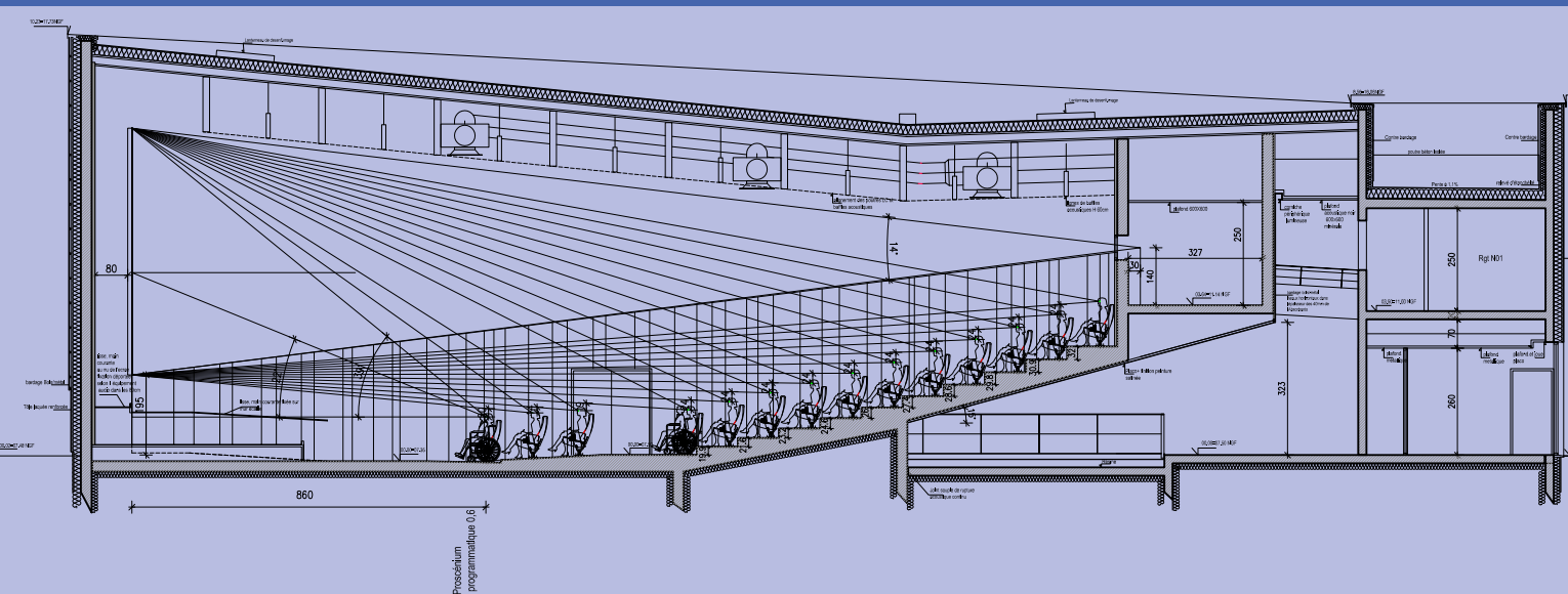
Coupe d'implantation et de visibilité, vue intérieure de la grande salle.
